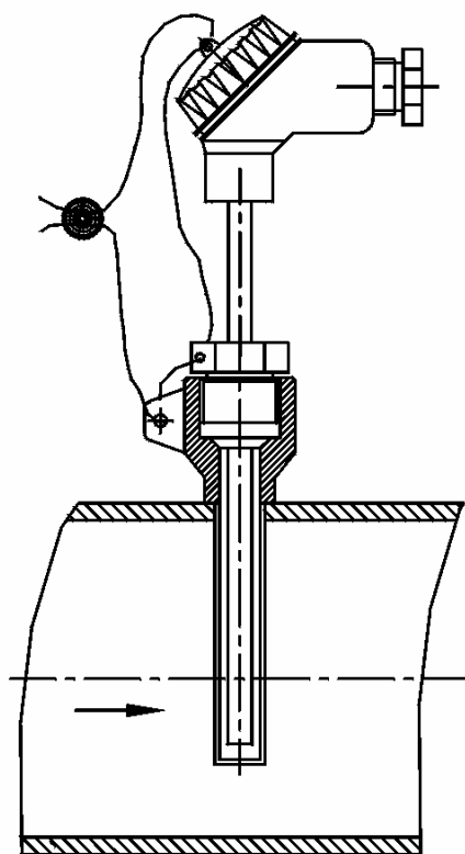
Рис 2. Схема монтажа термопреобразователя с защитной гильзой на трубопроводе (только для трубопровода D_u \ge 50 )
