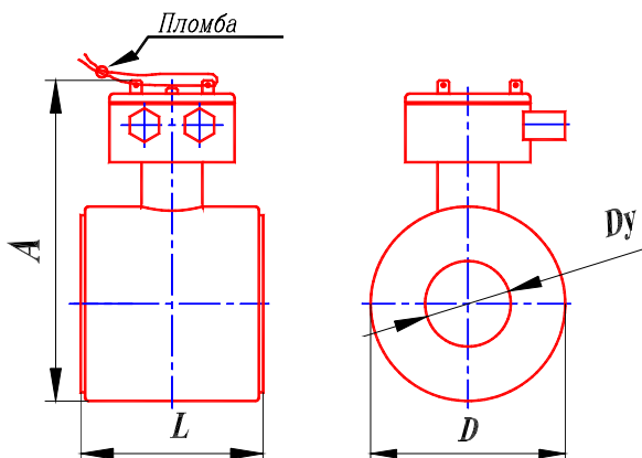
а) без монтажного комплекта
