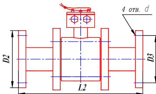
г) с фланцевым монтажным соединением (по EN 1434 – 2; 1998)
